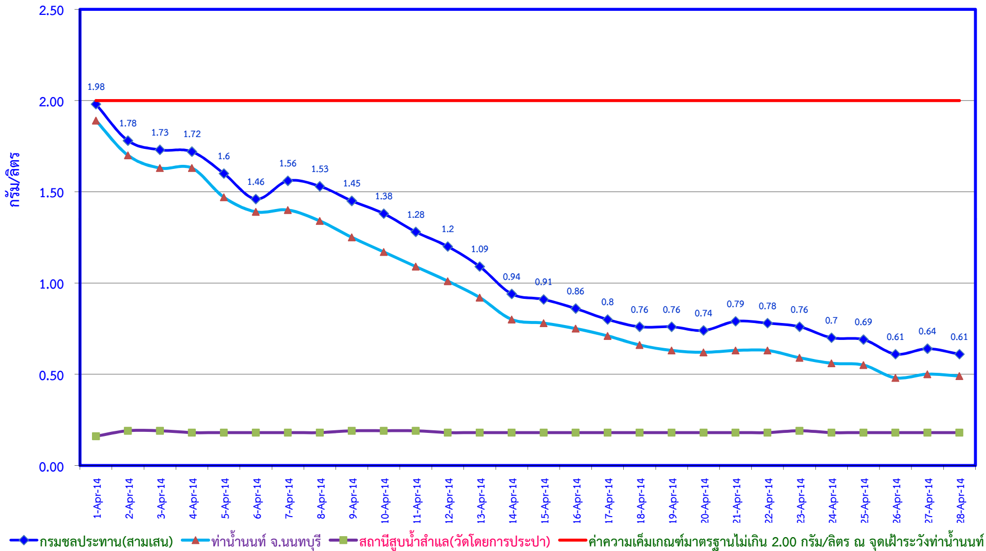
ค่าความเค็มแม่น้ำเจ้าพระยาที่กรมชลประทาน(สามเสน) ทำนํ้านนท์ และสถานีสูบน้ำประปาสำแล ประจำเดือนเมษายน ปี 2557
